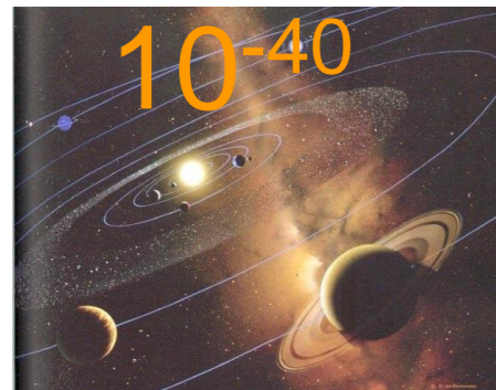
Forza gravitazionale
