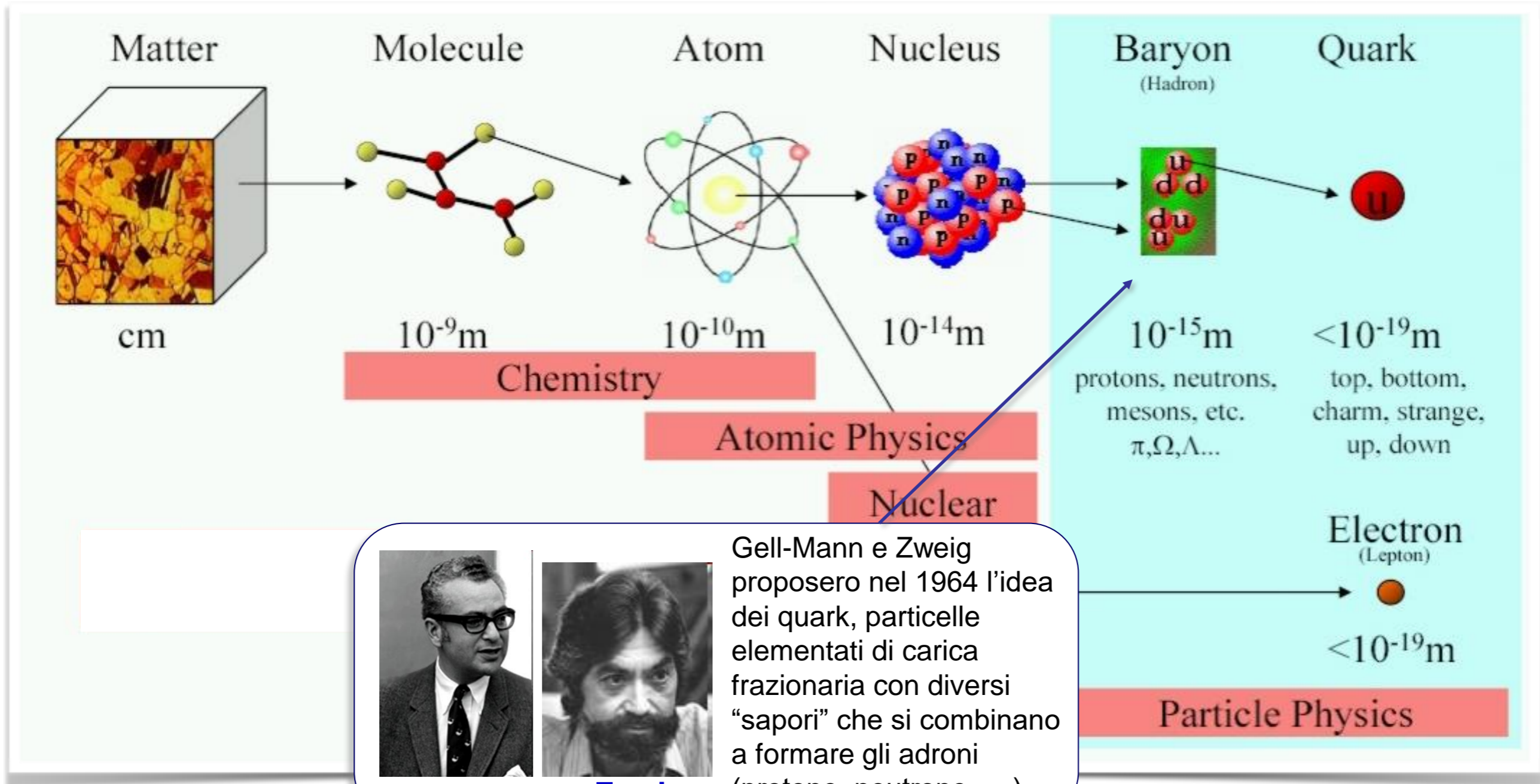
Gell-Mann
